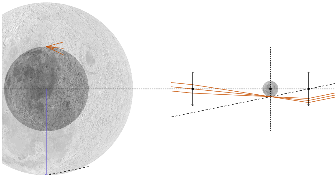
Obrázek 9: Náhled appletu chodu světelných paprsků v Keplerově dalekohledu. K dispozici online [3]. Zobrazený náhled neobsahuje ovládací prvky appletu. Paprsky jdoucí od krajního bodu se nám ve veliké vzdálenosti jeví jako rovnoběžné. Tyto paprsky se protínají v jediném bodě na ohniskové rovině, kde vzniká reálný obraz. Po průchodu okulárem získáme opět rovnoběžný svazek paprsků, který jde do našeho oka. Přerušovaná čára znázorňuje pozorovaný zdánlivý obraz okuláru, který je zvětšený oproti pozorovanému předmětu.
